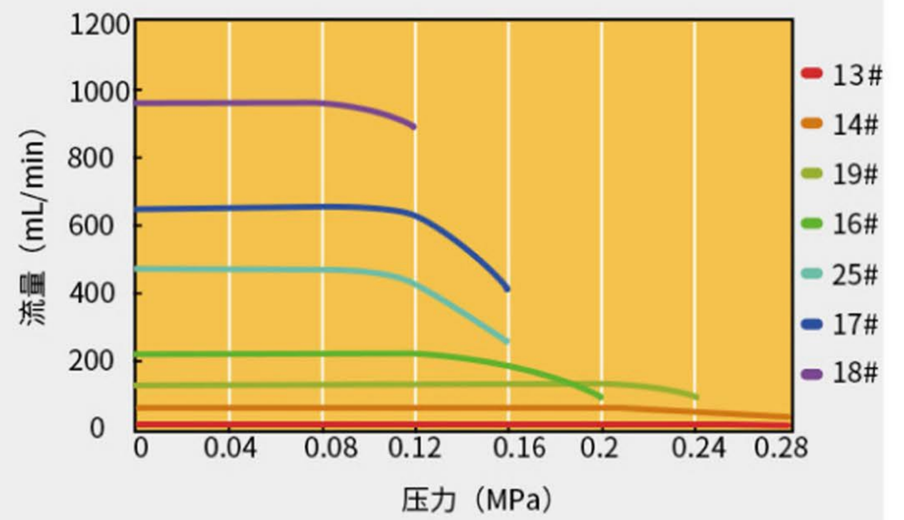
DY15泵头压力/流量曲线图 (100rpm)
